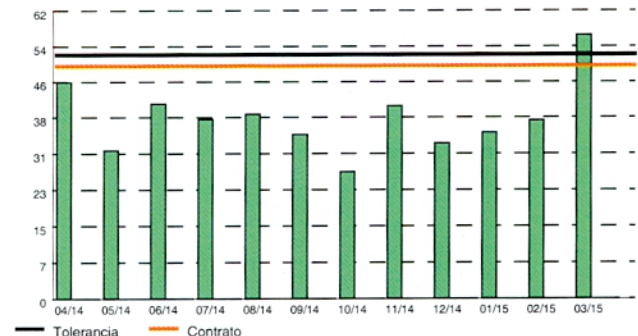
Demanda (kW)
