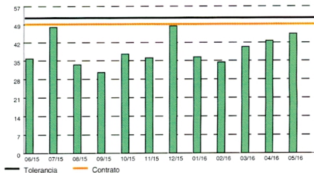
Demanda (kW)
