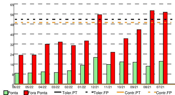
Demanda (kW)
